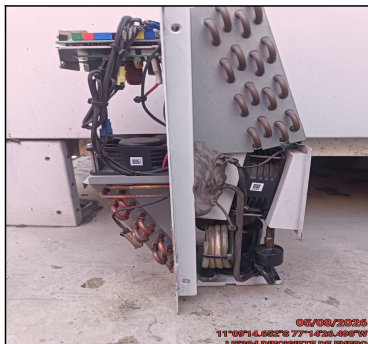
FOTO PANORAMICA DE TUBERIAS DE ALTA Y BAJA
