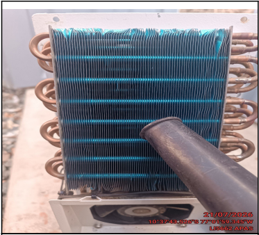
FOTO LIMPIEZA Y ESTADO DE SERPENTIN DE UC
