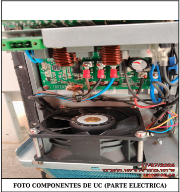
FOTO COMPONENTES DE UC (PARTE ELECTRICA)
