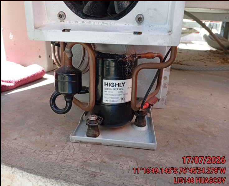
FOTO 8: REVISIÓN DEL COMPRESOR
