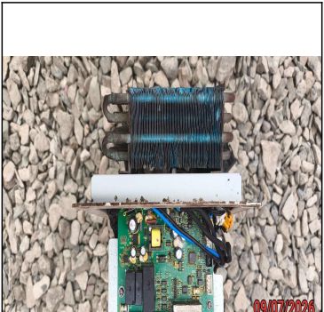
FOTO DE COMPONENTES DE UE (PARTE ELECTRICA)
