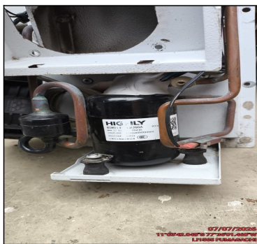
FOTO CORRIENTE REAL EN COMPRESOR
