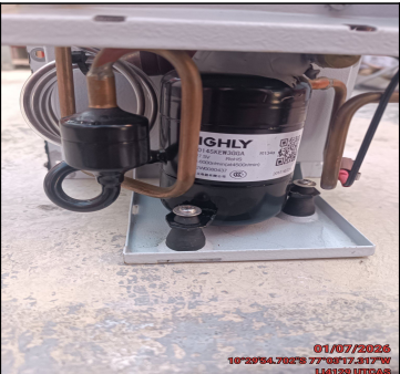
FOTO CORRIENTE SEGUN PLACA COMPRESOR
