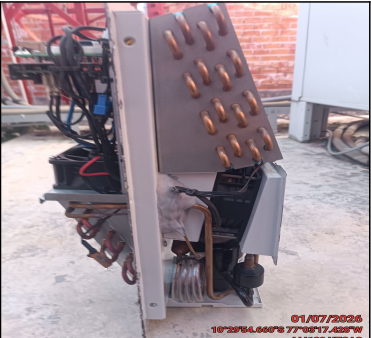
FOTO PANORAMICA DE TUBERIAS DE ALTA Y BAJA
