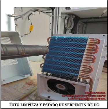
FOTO LIMPIEZA Y ESTADO DE SERPENTIN DE UC
