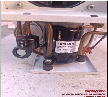
FOTO CORRIENTE REAL EN COMPRESOR
