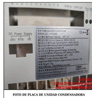
FOTO DE PLACA DE UNIDAD CONDENSADORA
