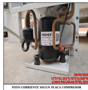
FOTO CORRIENTE SEGUN PLACA COMPRESOR
